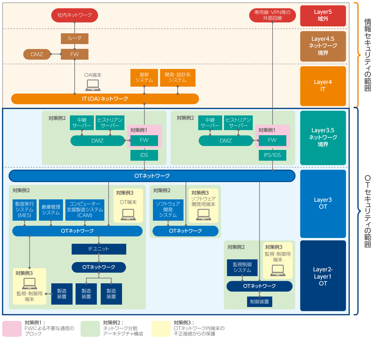
Purdue参照モデルをベースにした工場システムの全体像概要
