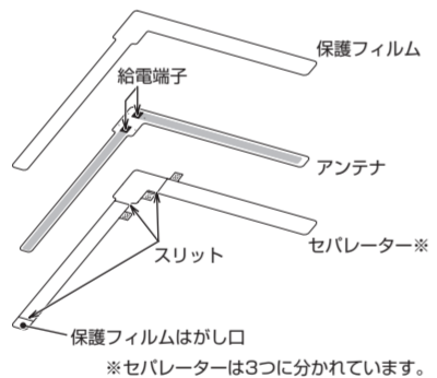
TV アンテナ (B) の構成
