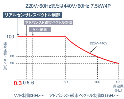
SF-PR-VSインバータ組合せ特性 ※代表値(参考値)
