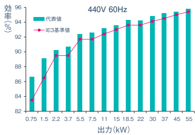
SF-PR-VS (4P)の効率 ※代表値(参考値)
