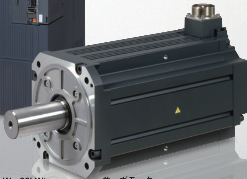
サーボモータ HG-JRシリーズ (200V/400V仕様 11kW~22kW)
