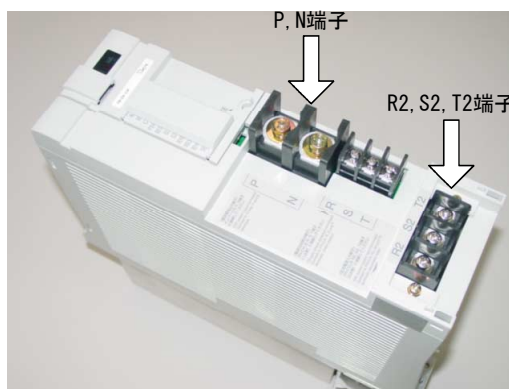
配線カバーを取外した状態
