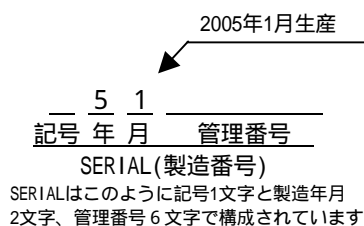
定格銘板例
