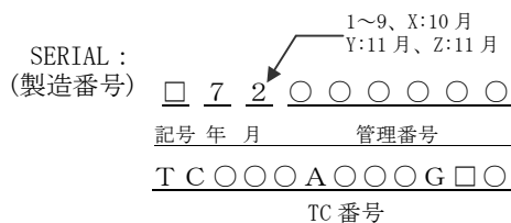
定格名板例
