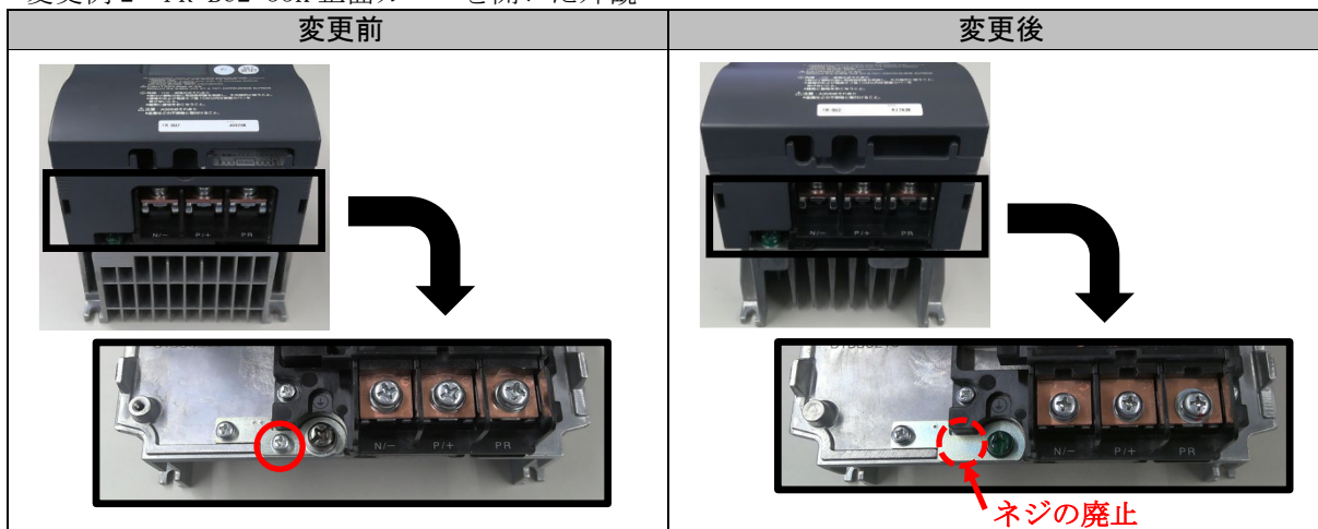
変更例2 FR-BU2-55K 正面カバーを開いた外観
