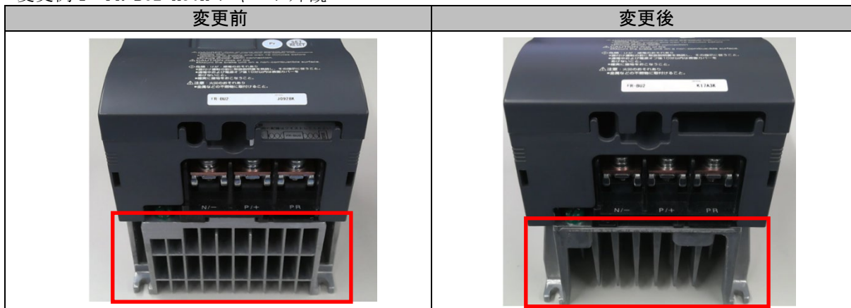
変更例1 FR-BU2-H30K シャーシ外観
