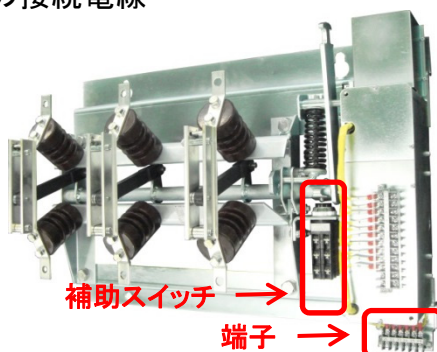
図 1. DV-HM形補助スイッチ／端子間の接続電線部
