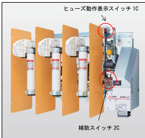
図 1. 変更対象部位(代表機種TES-GB1)
