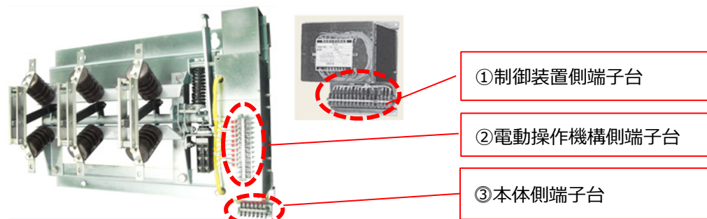
図 1. 外観及び変更箇所 (代表例：DV-HM 形)
