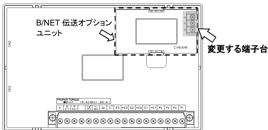
図 1 MP11A 背面図
