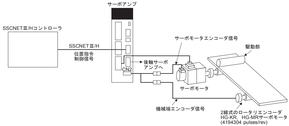
図1 システム構成 (MR-J4-Bサーボアンプの場合)
