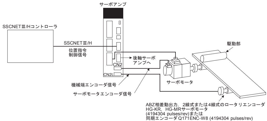
図2 システム構成 (MR-J4-B-RJサーボアンプの場合)
