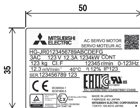
図4. 変更後の本体ラベル
