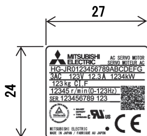
図3. 変更前の本体ラベル
