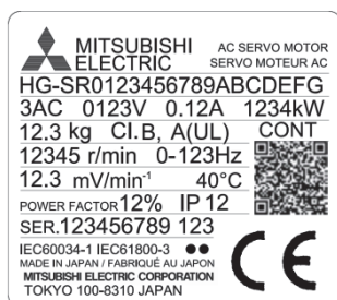
図1. サーボモータ本体ラベル印字例(名板2枚)
