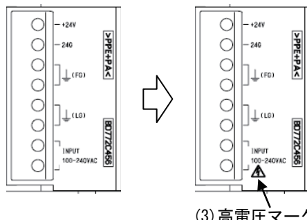
図2. 扉内側表示
