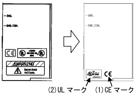
図1. 扉外側表示
