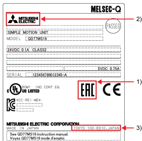
図1. 定格銘板表示例 (QD77MS16)
