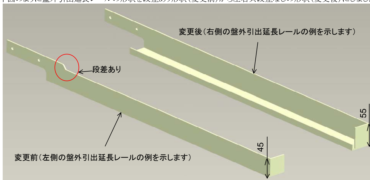
図 盤外引出延長レールの形状変更
