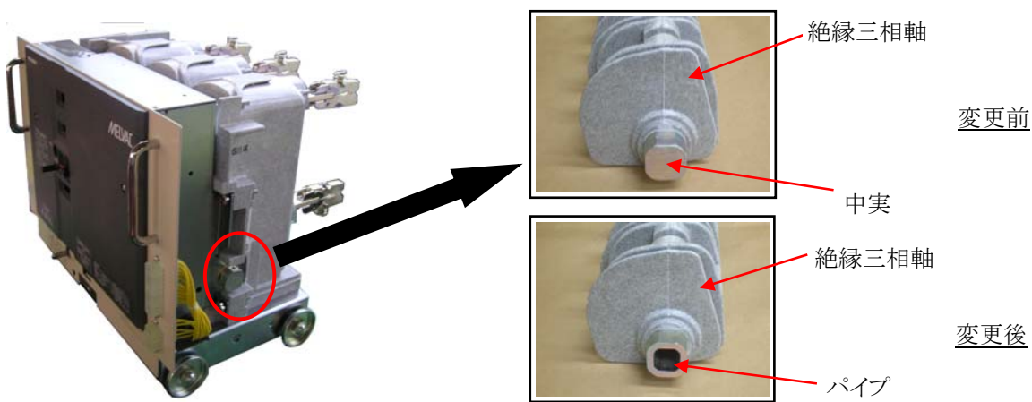
図 VF-8D/13D/8DBS/13DBS形VCB本体の軽量化
