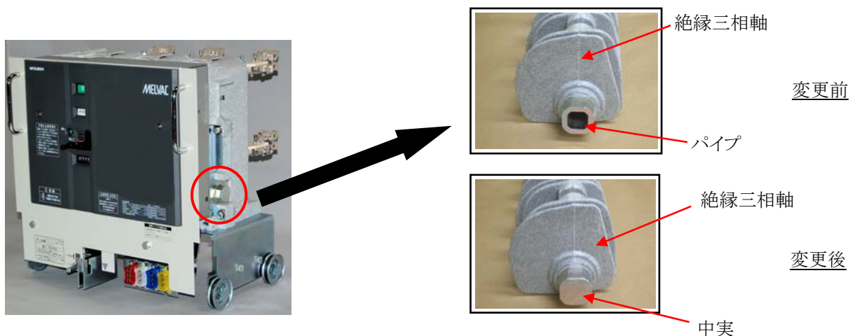
図 VF-8DA/13DA 形VCB本体の絶縁三相軸の変更の例
