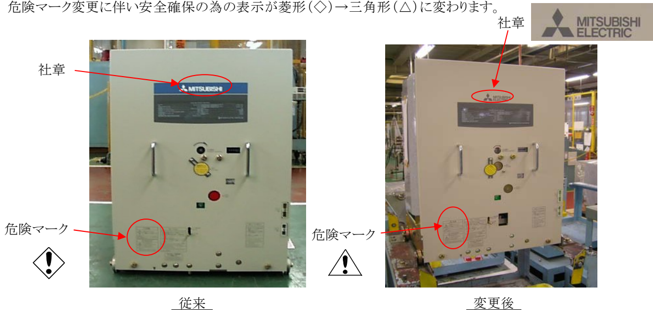
図 フェースプレートの変更前後(VF-32C/40C形VCBの例)
