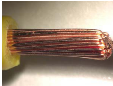
変更後(先端部の被服を剥いた状態)
