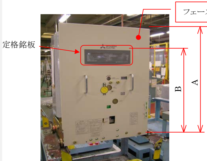
図 定格銘板の位置
