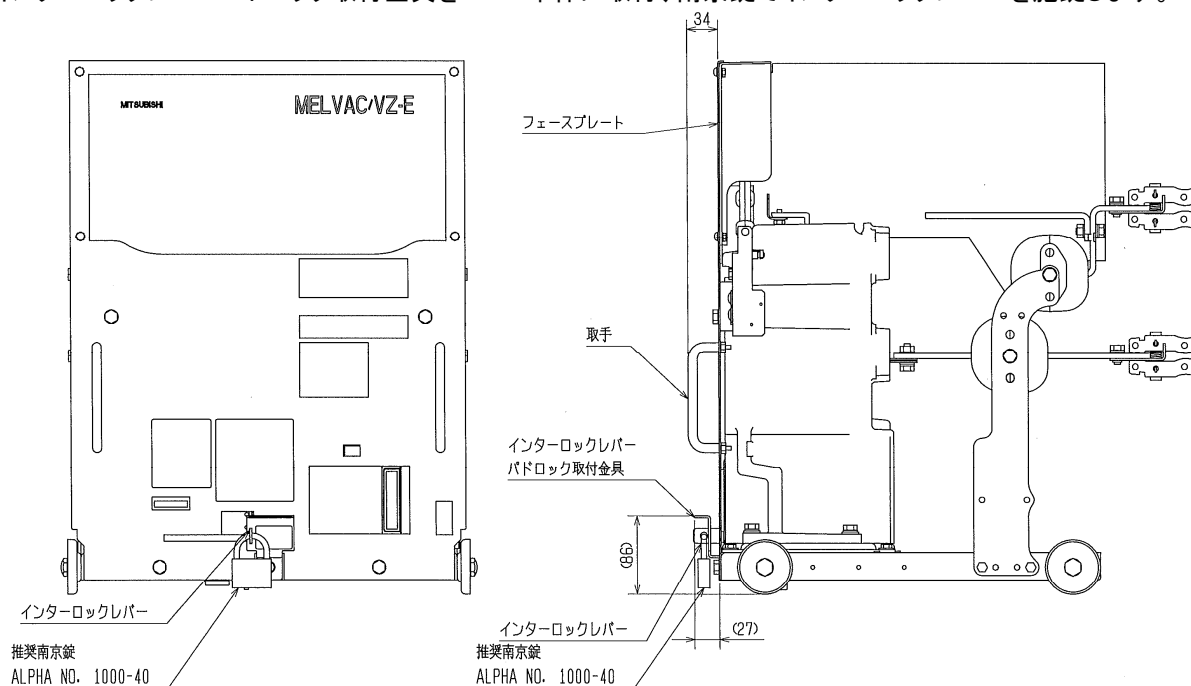
図1 インターロックレバーパドロック取付状態
