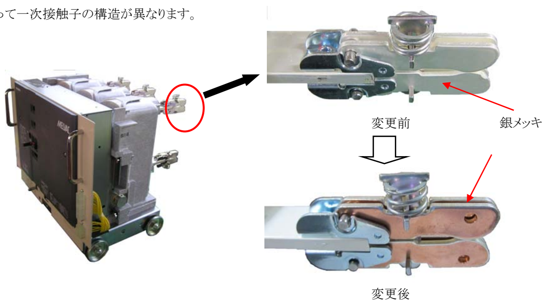
図 高圧真空遮断器 VF-8D/13D 形一次接触子の仕様変更例
