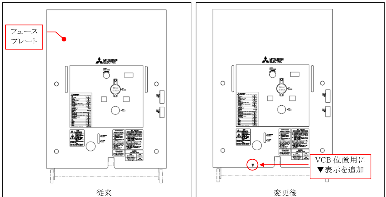
図 フェースプレートの変更前後(3/6/10/15-VPR-25D/32D/40D 形 VCB の例)
