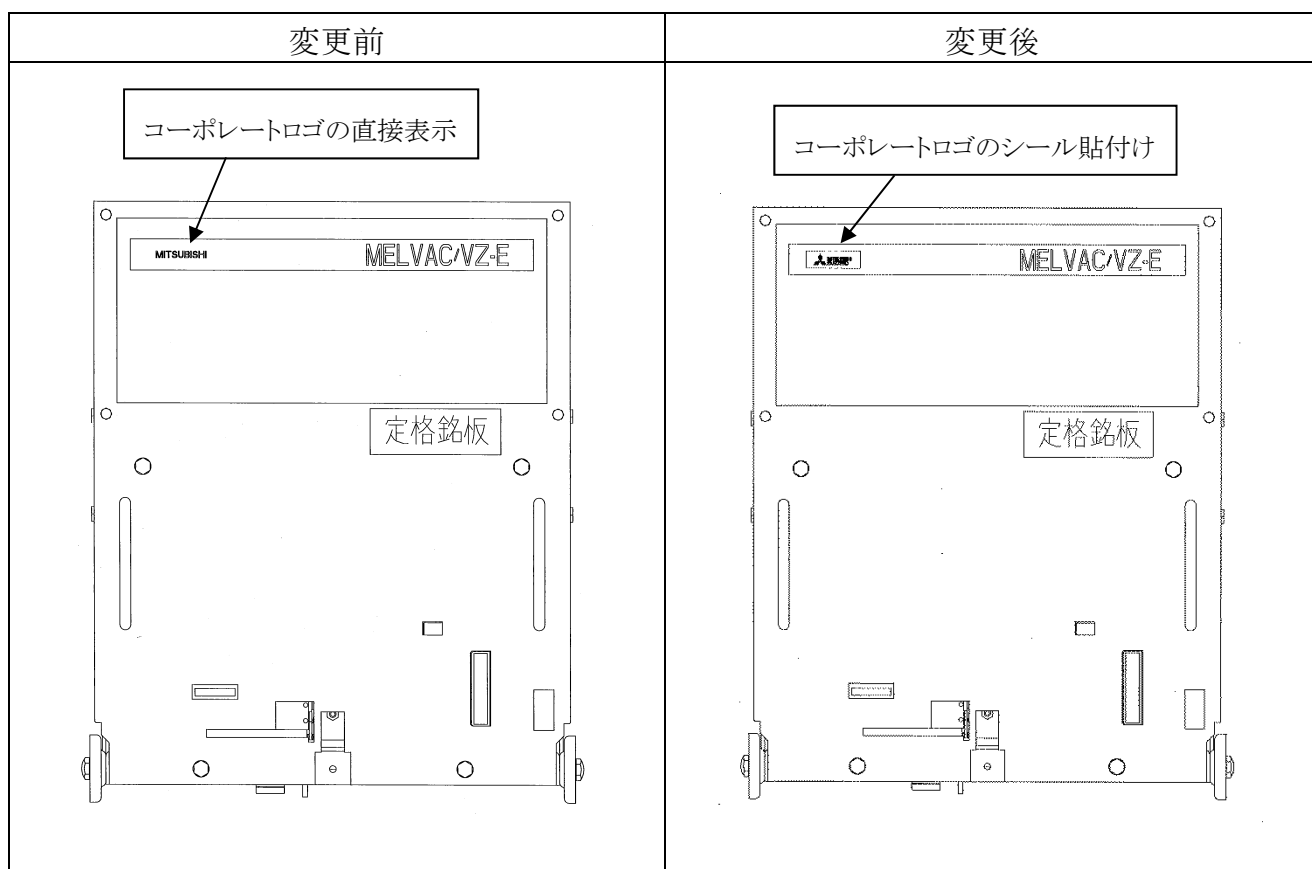
図4 代表例 3: 高圧真空電磁接触器 VZ-E シリーズ(フェースプレート)
