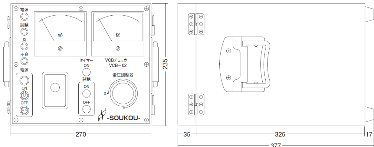
図 1 双興電機製作所製 VCB チェッカー外形図 ※VCB-02 を掲載(外形寸法は VCB-02, VCB-30 共に同一)
