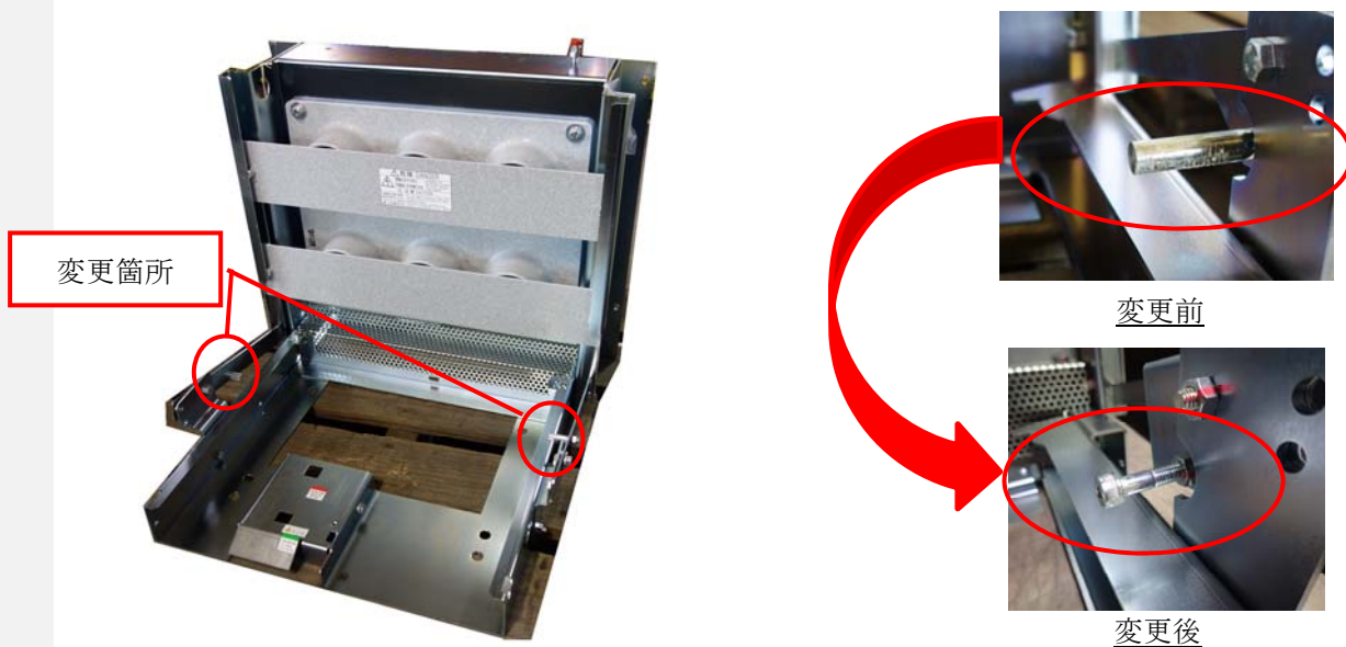
図 シャッター駆動レバーピン(PW/MW 固定枠)の変更前後
