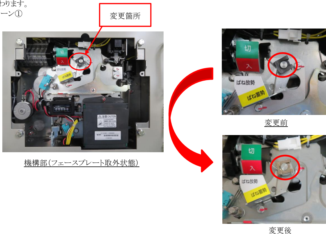
図1 止め輪の変更前後(パターン①)
