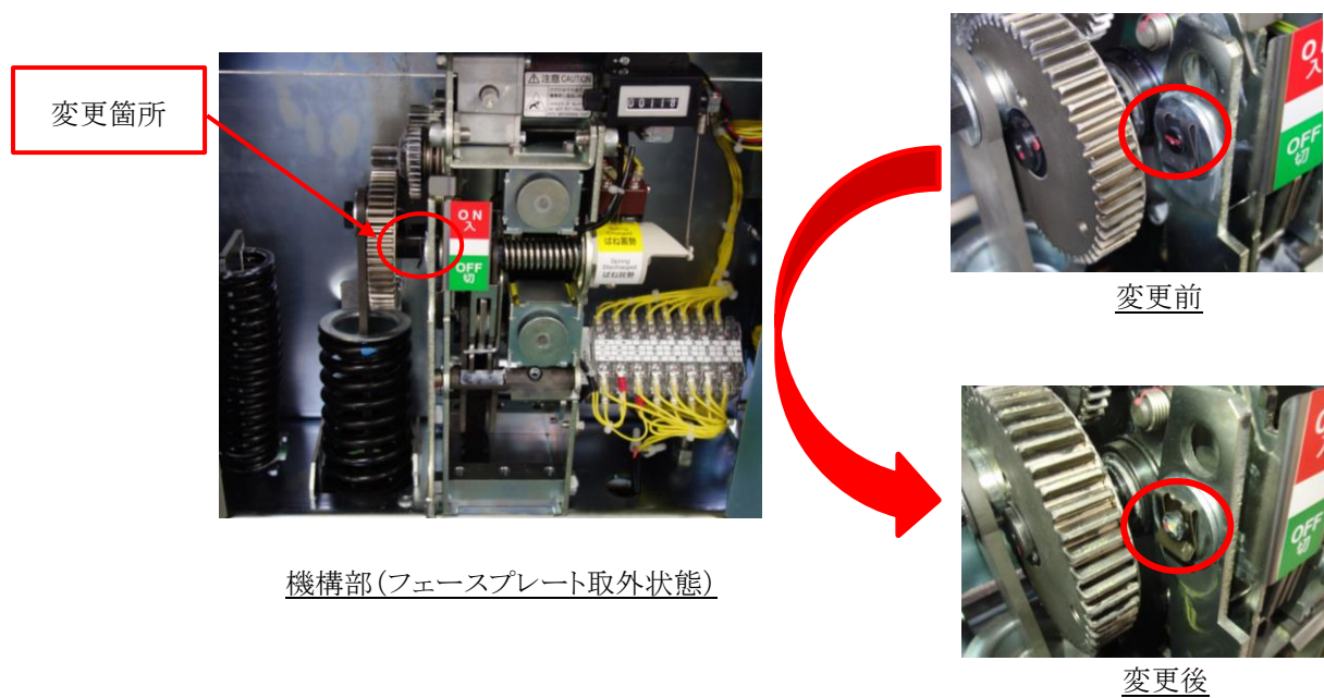
図2 止め輪の変更前後(パターン②)
