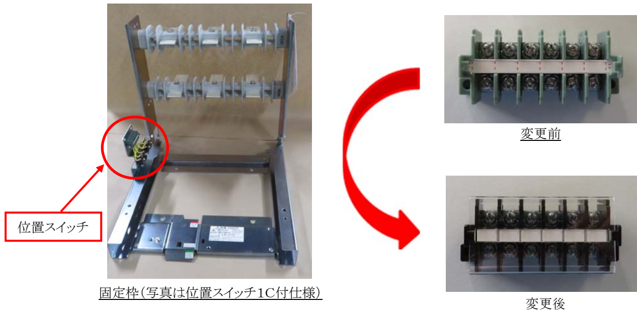
図1 位置スイッチ端子台の変更前後
