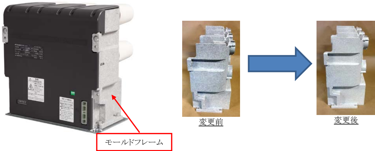
本体(写真は真空コンタクタ固定形)
