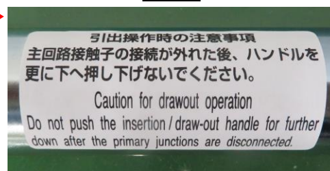
図2 挿入ハンドル銘板変更前後
