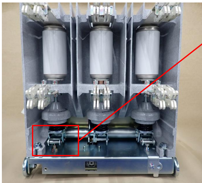
図1. 遮断器背面
