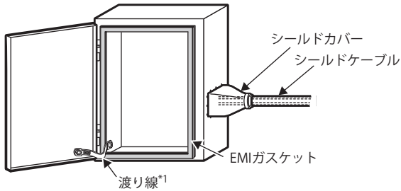
図2 制御盤の製作例
