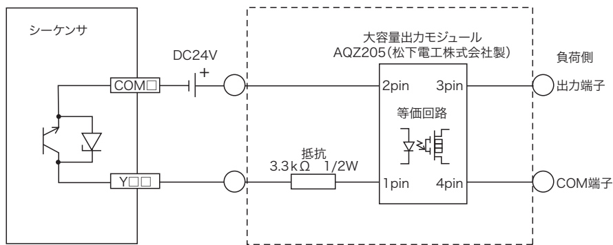
『代替回路 (参考図)』
