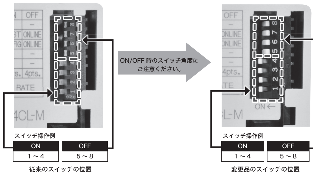
FX2N-64CL-M のトップカバーをはずしたスイッチ部分
