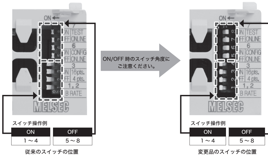
FX3UC-32MT-LT のディスプレイモジュールをはずしたスイッチ部分
