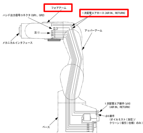
ハンド用配線・配管形態
