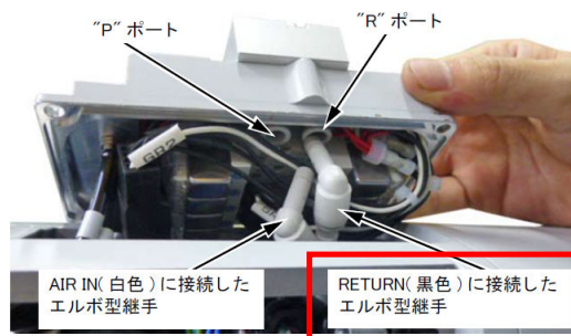
電磁弁セット取付け写真
