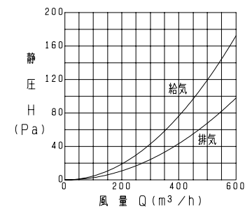
P-18VA 2 圧力損失特性
