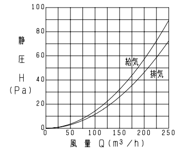
P-13VA 2 圧力損失特性
