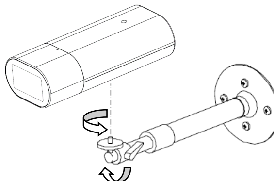
図 8-2 標準据付工事方法
