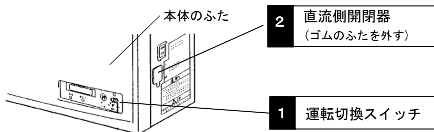
パワーコンディショナ操作部
