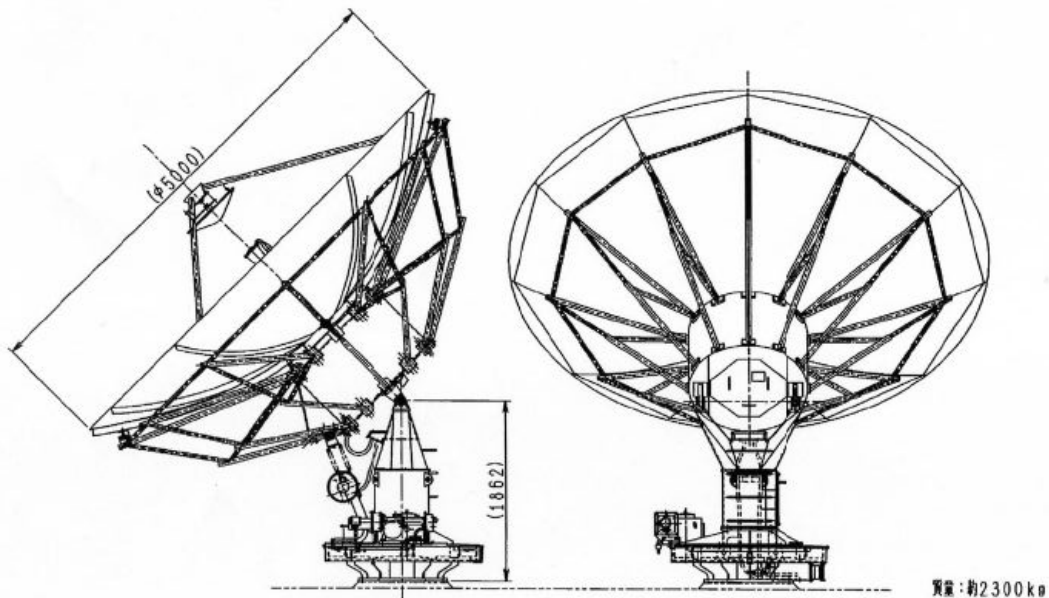
5mφ汎用受信アンテナ外観図
