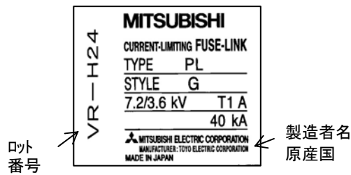
<一次側ヒューズの定格名板表示>
