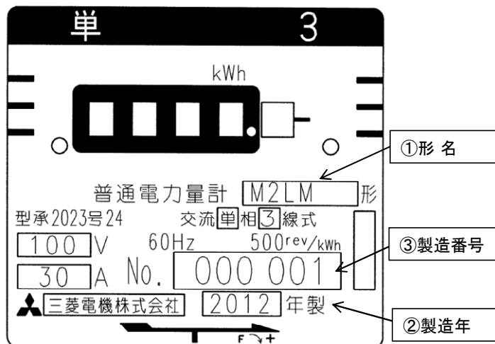
本体定格銘板図
