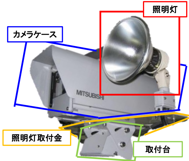
図1 組合せ型カメラ装置の構成・外観例(正面)
