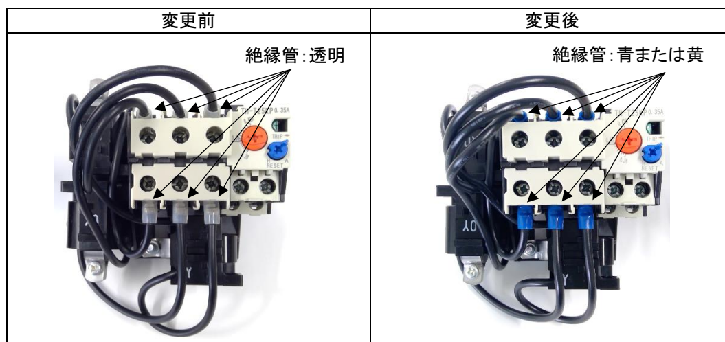
※写真は TH-T25KPSR 0.35A 形 サーマルリレーの場合を示します。
