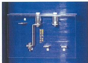
タップ切換部保護カバー(無色透明)
