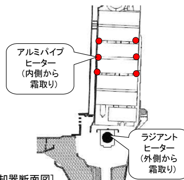
[冷却器断面図] 図 4 ハイブリッドデフロストヒーター
