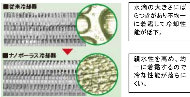
図 3 ナノポーラス冷却器 (従来冷却器との着霜比較)
