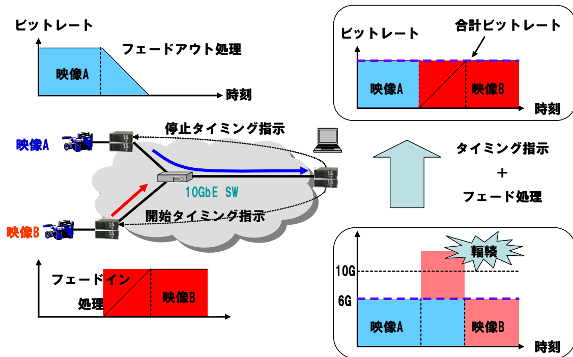
(図 3) 非圧縮 4K 映像素材をネットワーク上で切替編集する技術の概要
