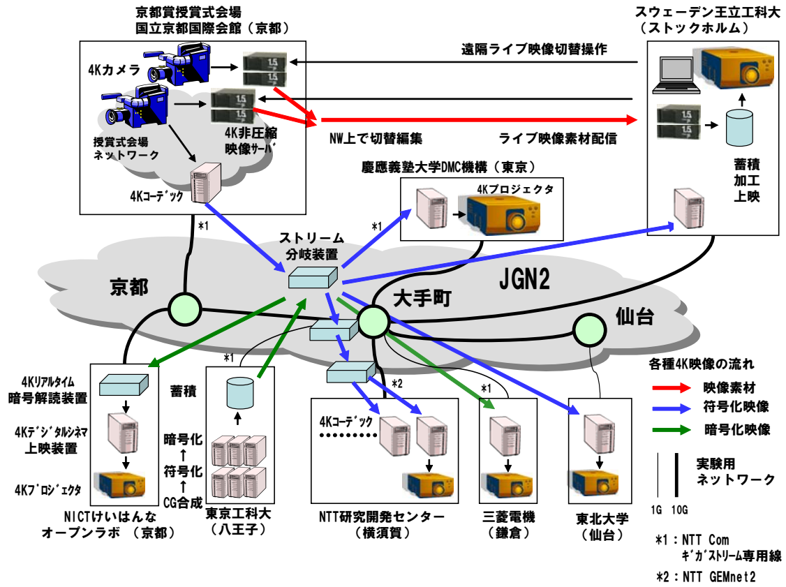
(図 1) 4K リアルタイム映像制作配信ネットワーク実験の概要
