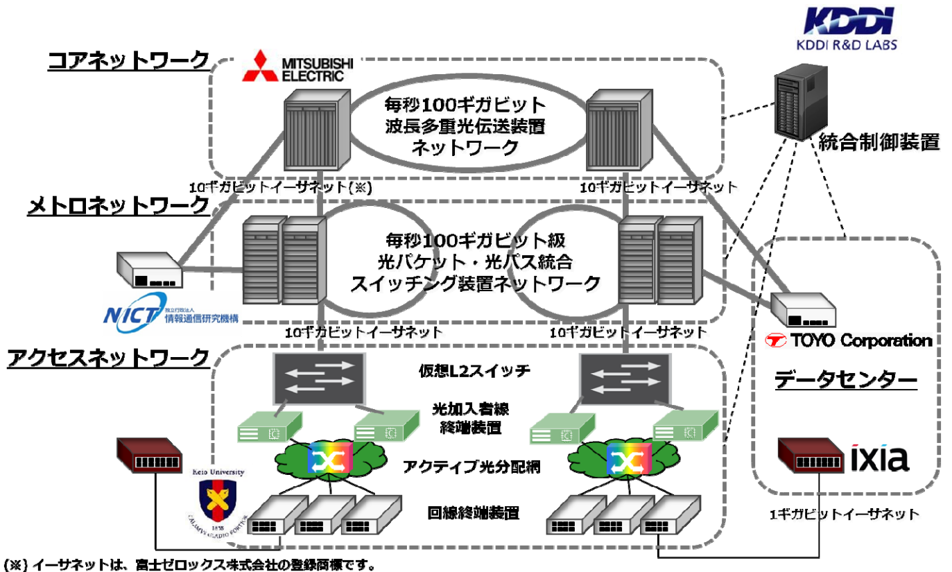
図1 データセンター間を接続する光ネットワーク構成
